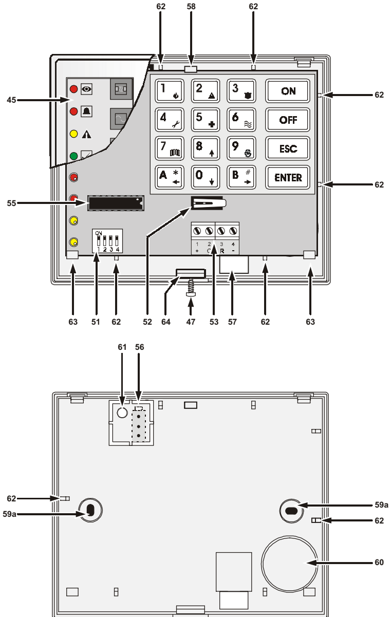
Fig. 1.3 - Tastiera NC2/TAST
