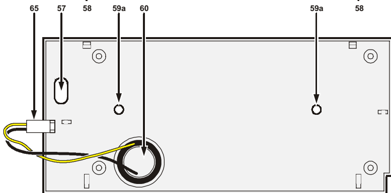
Fig. 1.4 - Tastiera ICON/KP
